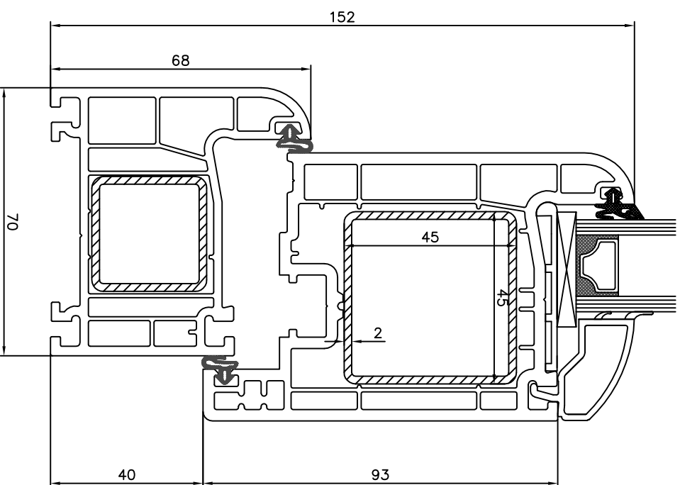
Rama 7010 + skrzydło 10001 + listwa przyszybowa 7030
