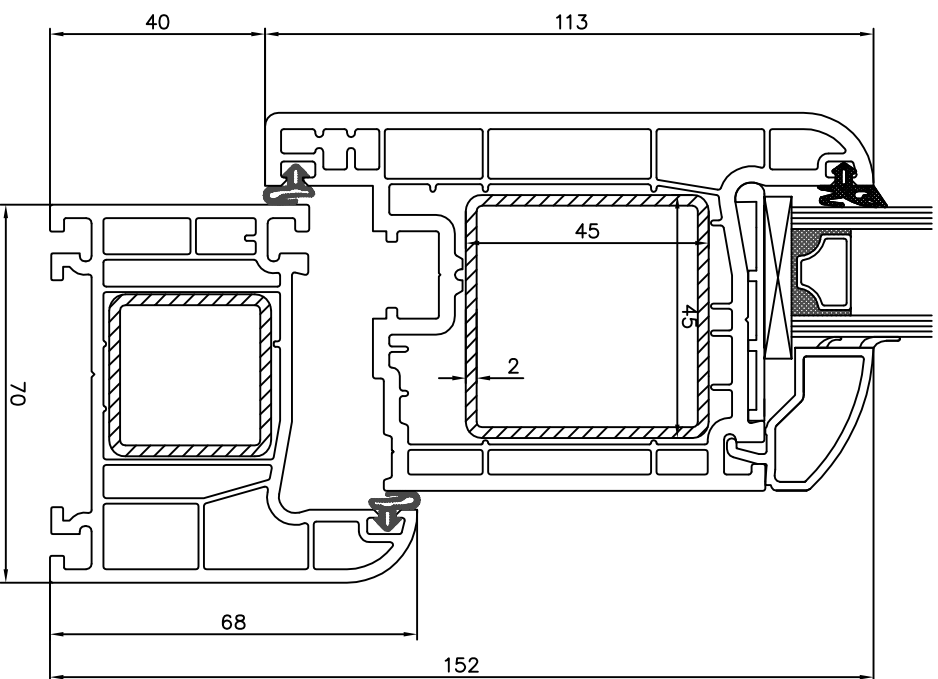
Rama 7010 + skrzydło 10002 + listwa przyszybowa 7030
